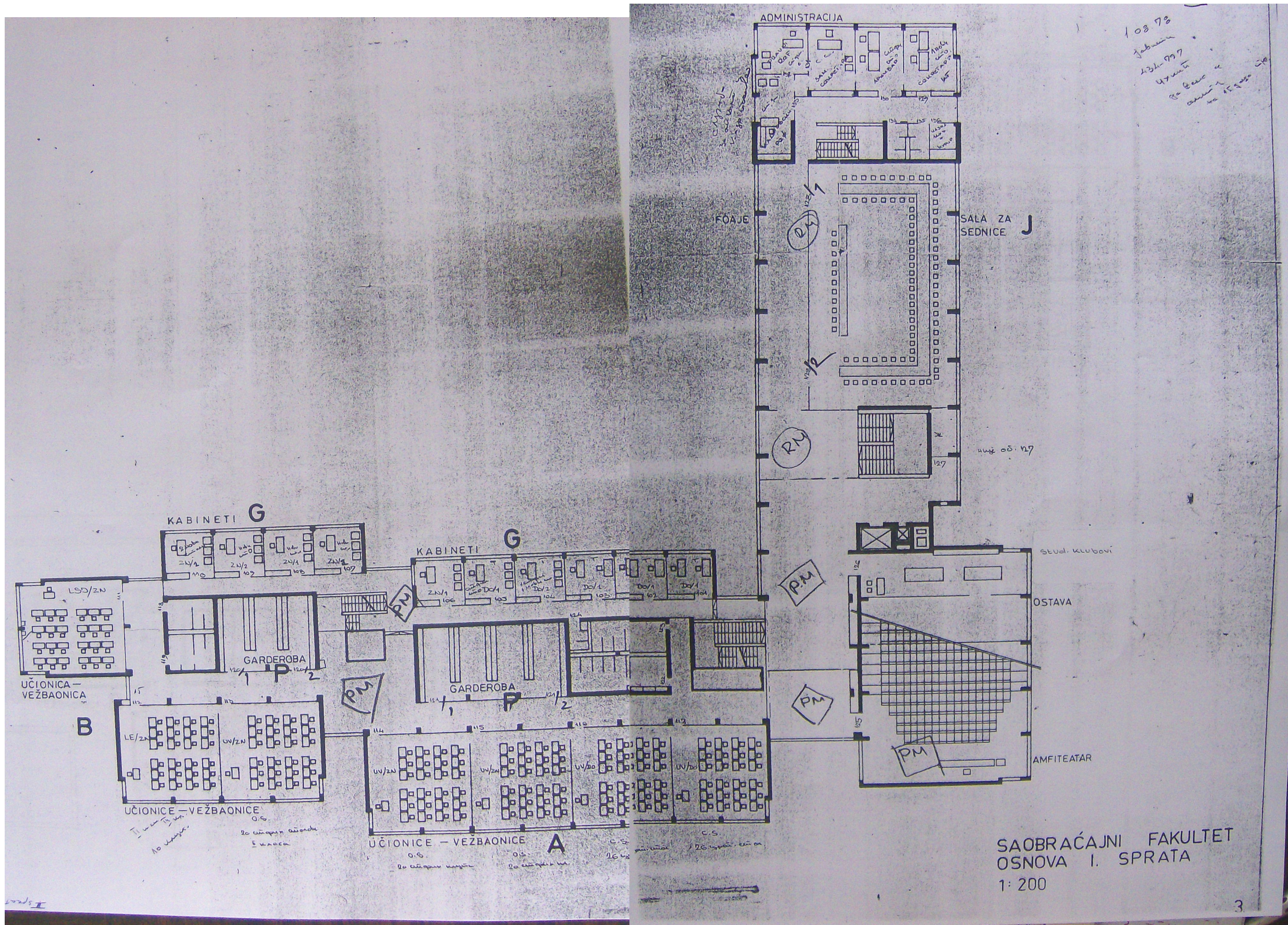
PLAN OSNOVE I sprata
