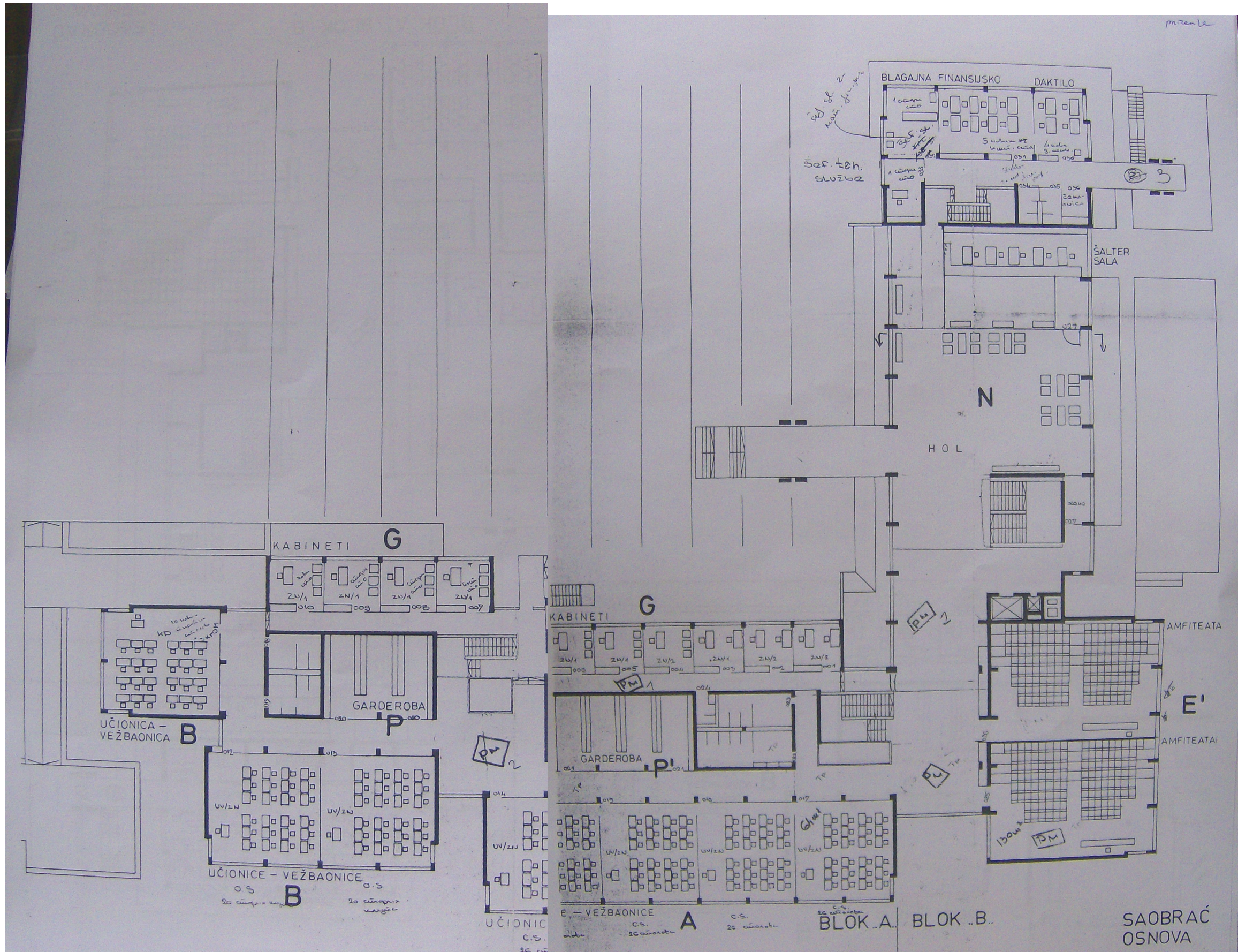
PLAN OSNOVE PRIZEMLJA
