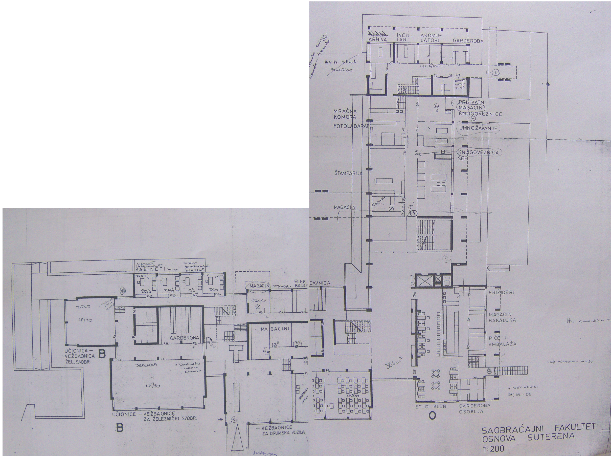
PLAN OSNOVE SUTERENA
